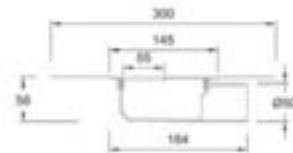
F-150K İzolasyon Kiti Isolation Kit
