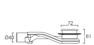
360° Döner Sifon 360° Rotate Siphon
