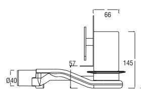
360° Döner Sifon 360° Rotate Siphon Ø40 / Ø50
